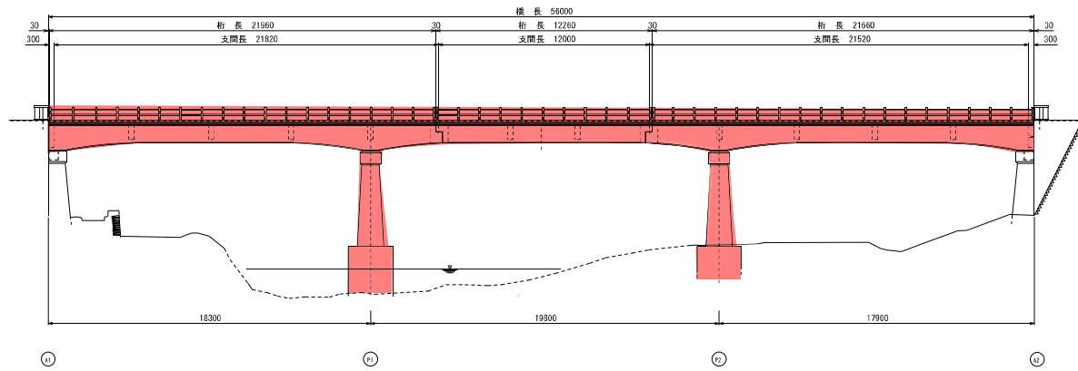
側面図 S=1:100
