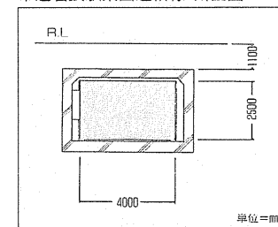
市道名張駅東西連絡線 断面図
