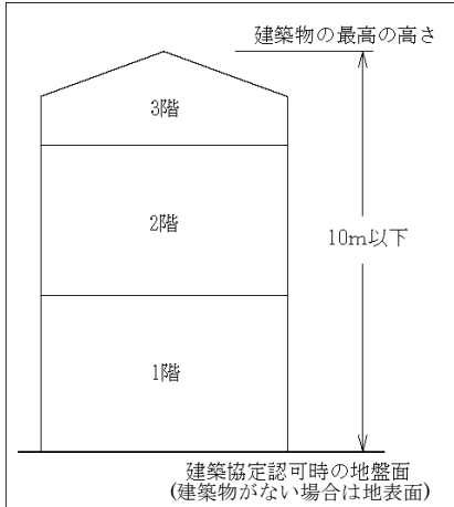
▼参考図① 建築物の最高の高さ
