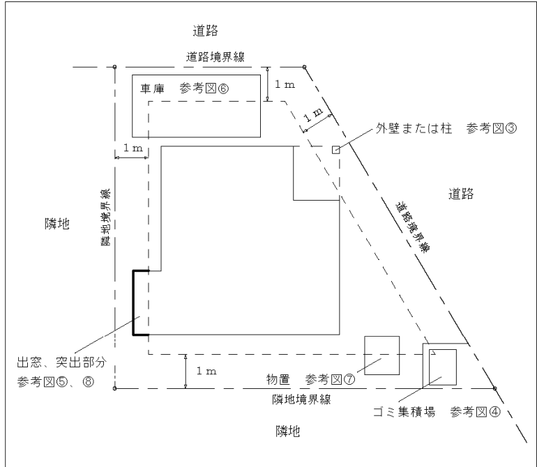
▼参考図② 道路境界線及び隣地境界線からの水平距離
