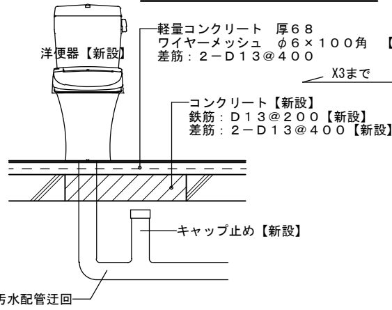
断面図 S = 1 / 3 0
