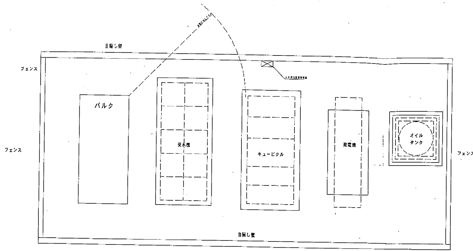
バルクタンク廻り平面詳細図 1/50
