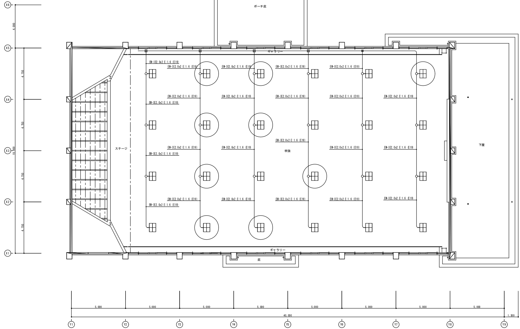
既設照明設備 平面図 S-1/NON
