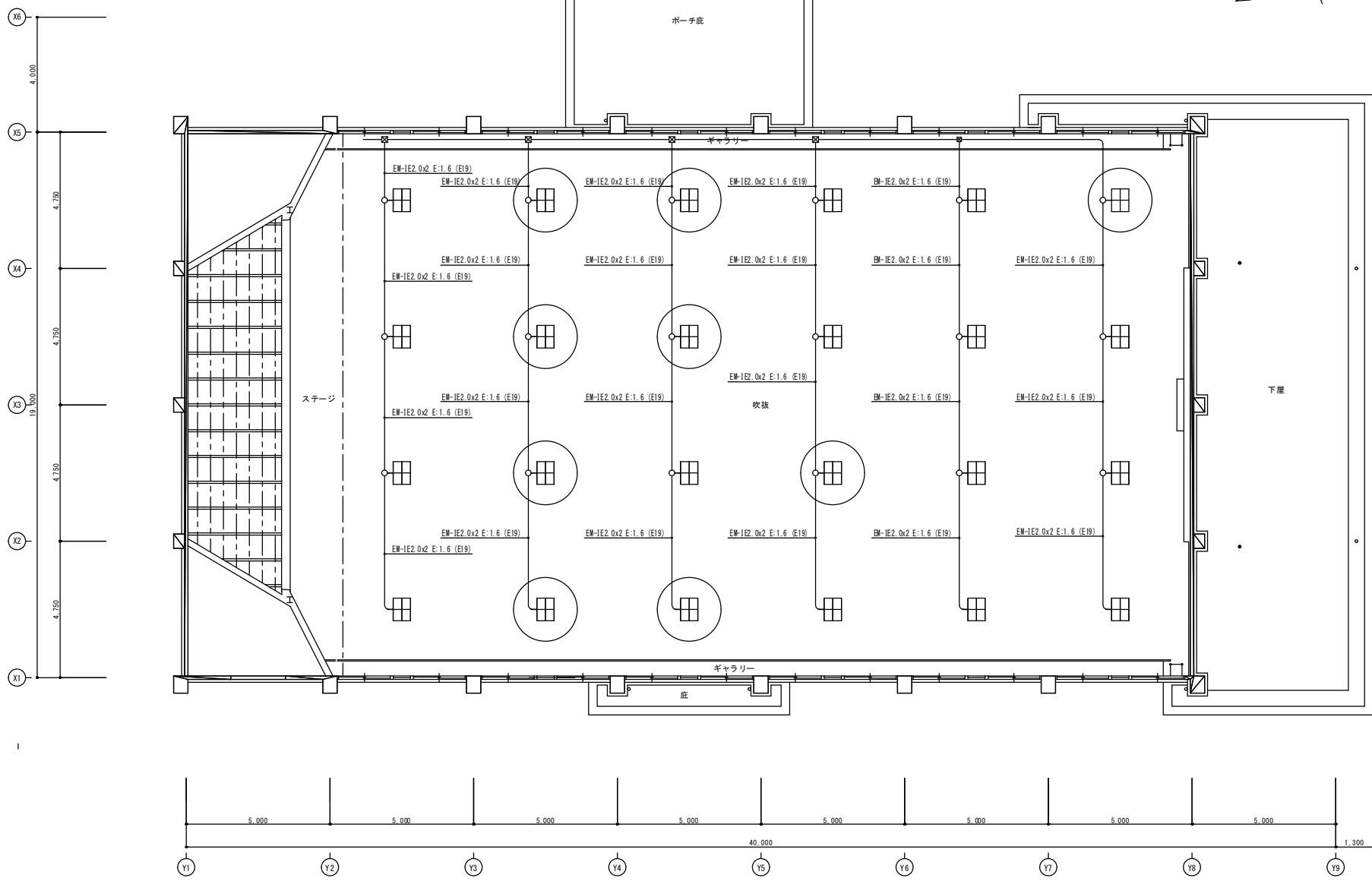
改修後照明設備 平面図 S=1/NON
