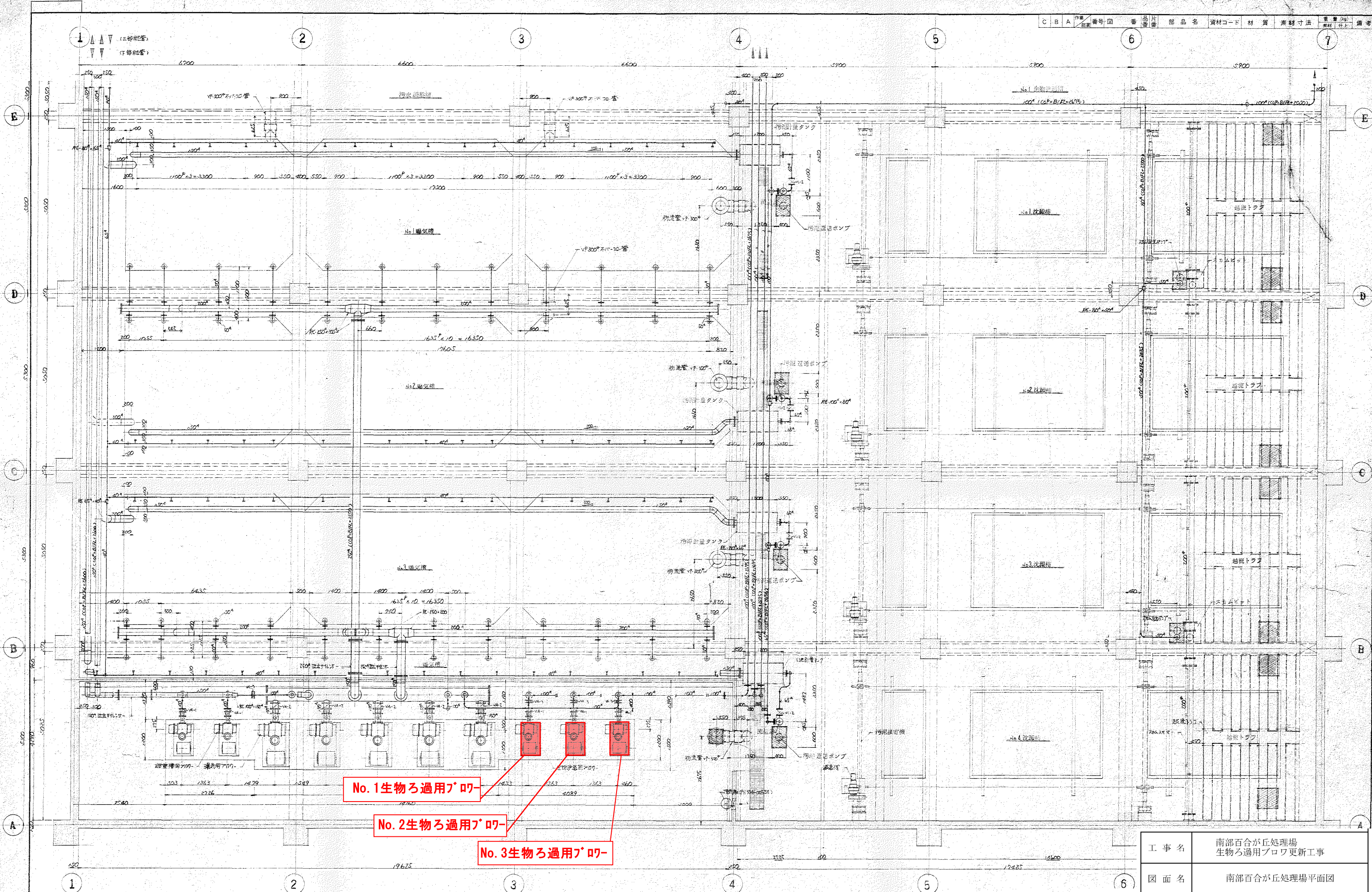
平面図 1:50
