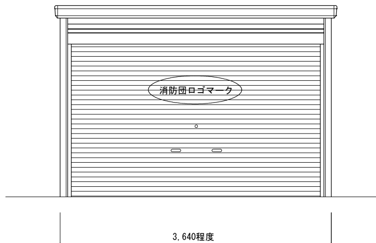
正面図 : 1/50
