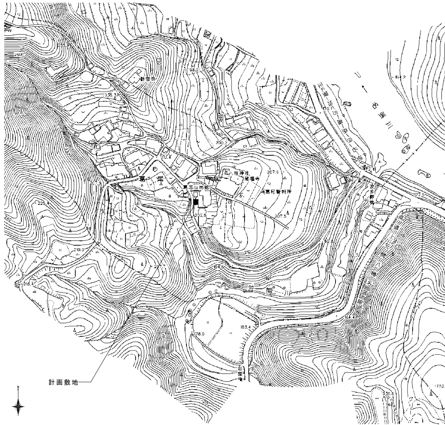
配置図：NS
