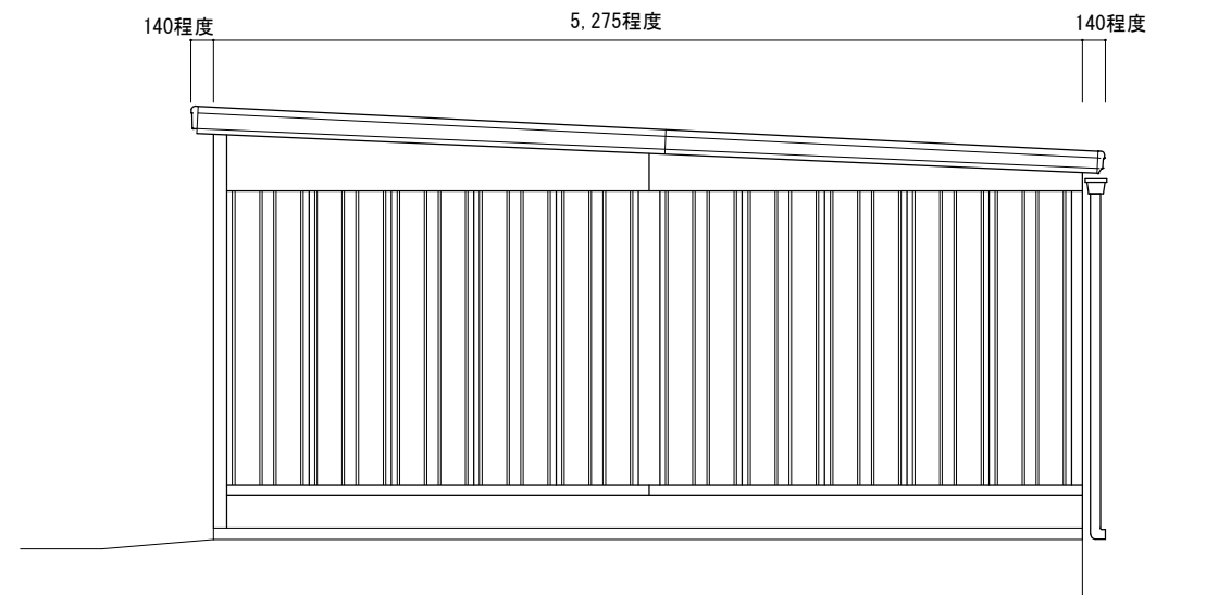
側面図 : 1/50
