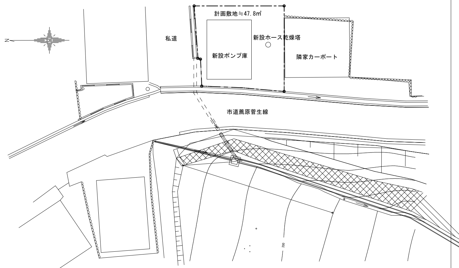
整備後(参考)：1/200
