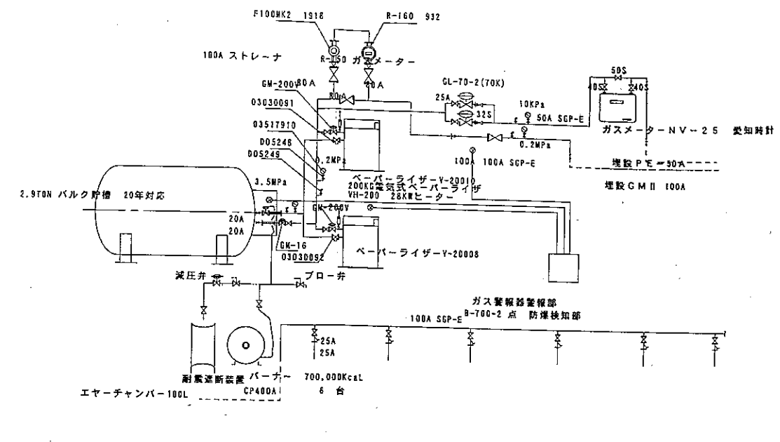
LPG 配管フロシート S=FREE
