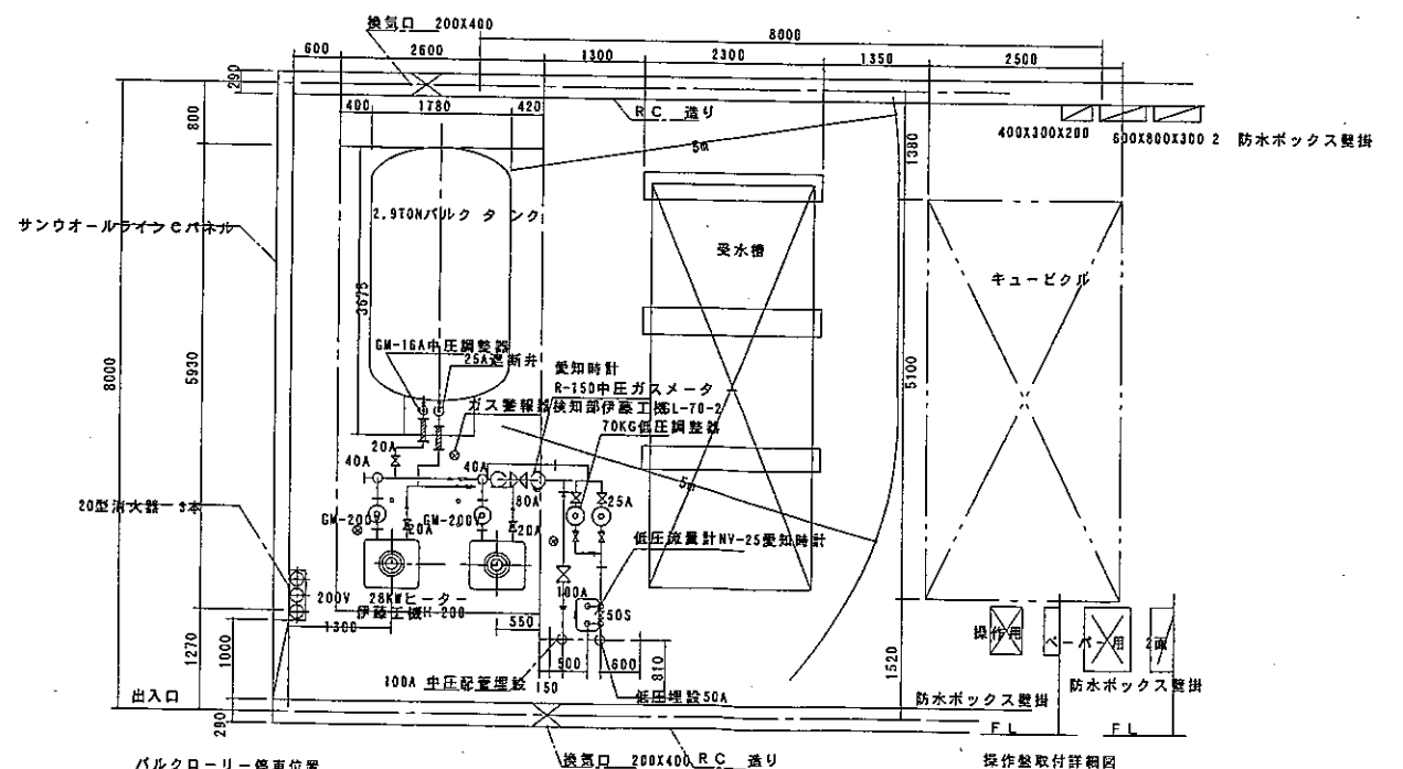
LPGバルク貯槽設備配管図 S=FREE
