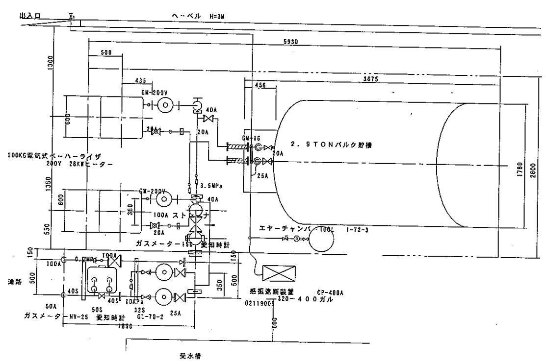
名張市斎場 LPG 配管系統図 S=FREE
