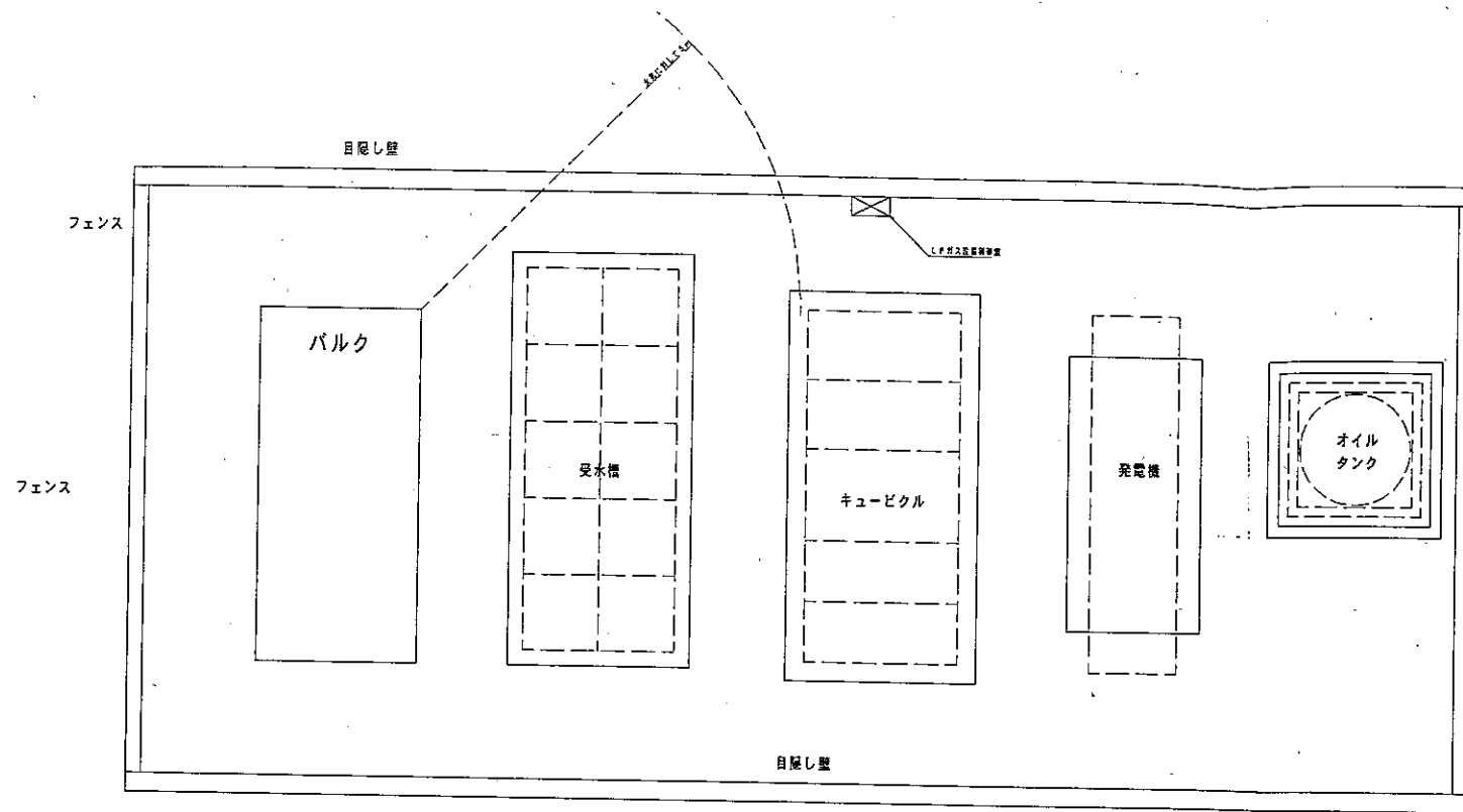
バルクタンク廻り平面詳細図 1/50
