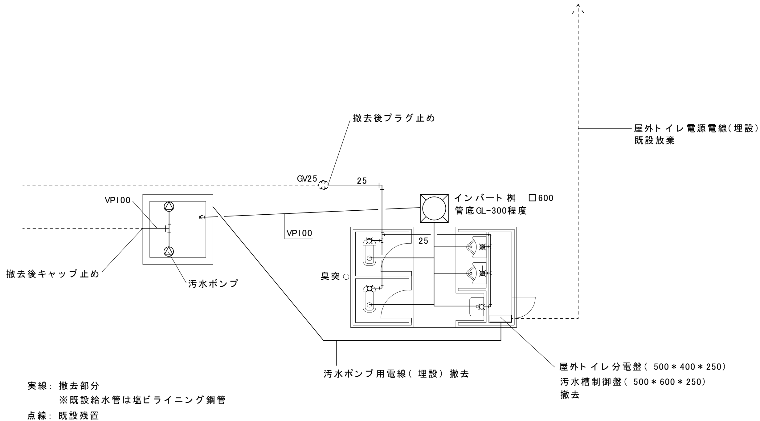
給排水衛生設備図兼電気設備図 1/50
