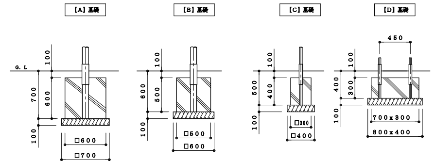
基礎詳細図 S=1/40
