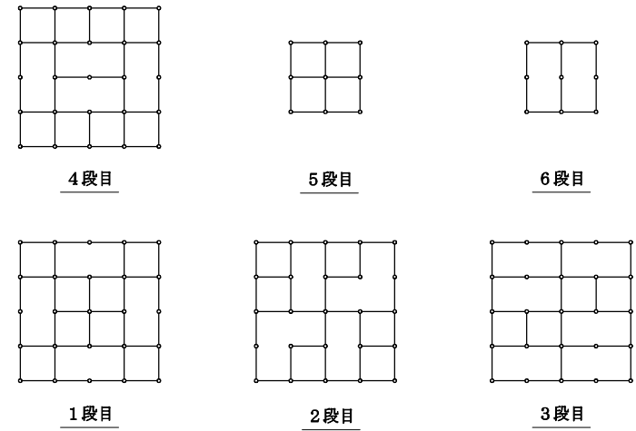
各段平面図 S=1/60
