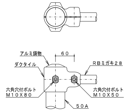
A詳細図 S=1/5
