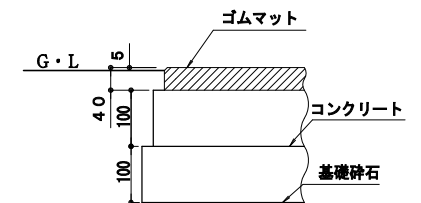
セーフティマット共通断面図 S=1/10
