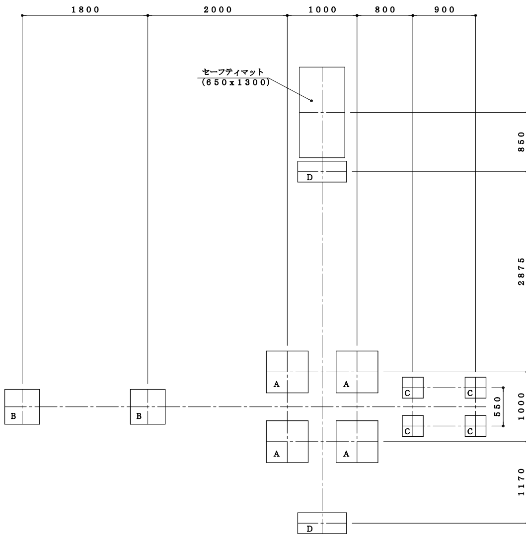
基礎伏図
