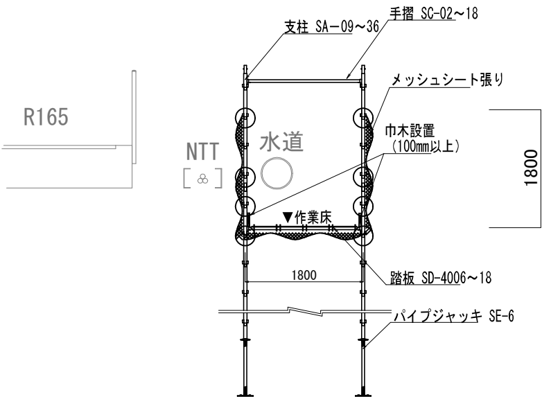
仮設断面図 S=1:Non
