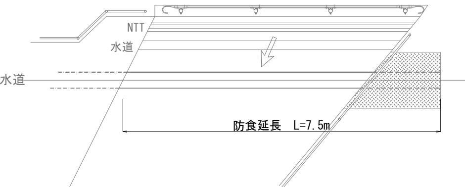
防食保護工側面図 S=1:Non
