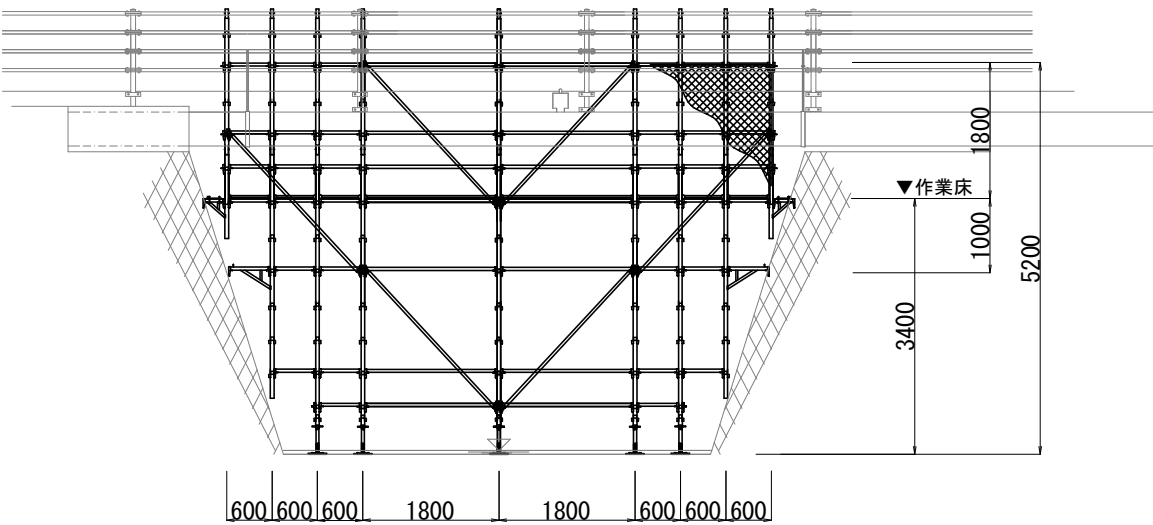
仮設断面図 S=1:Non
