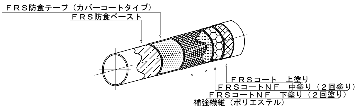
防食保護工工法図 S=1:Non
