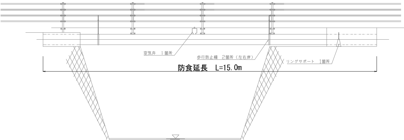
防食保護工工法図 S=1:Non
