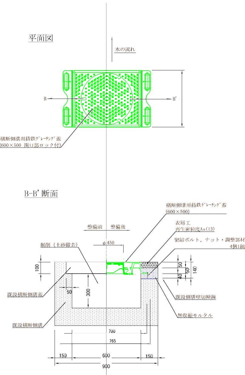
<側溝蓋②>
