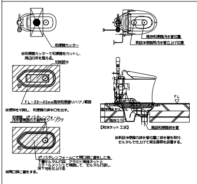
和洋改修工法参考図 参考工法：LIXILネット工法
