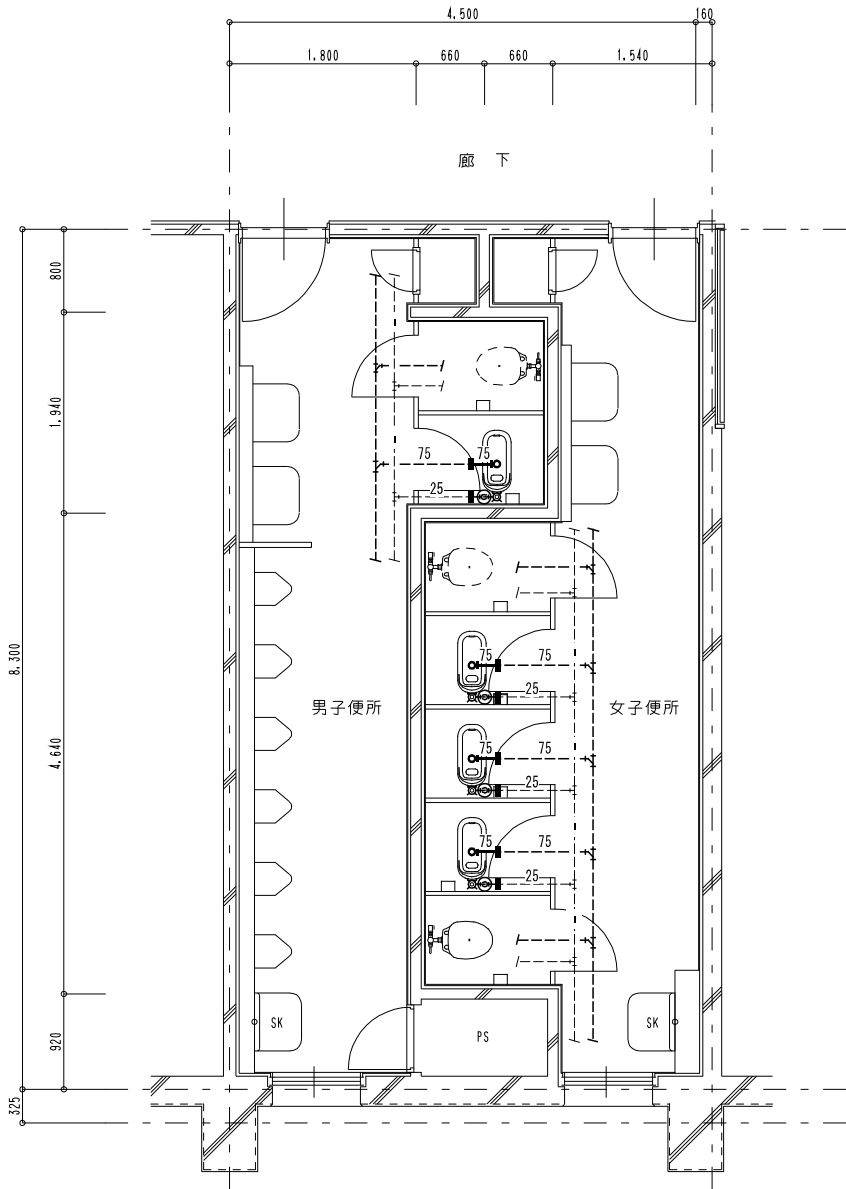
男子便所 既存機器表
