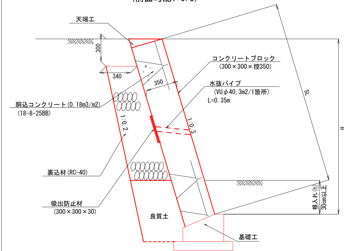
ブロック積標準断面図 S=1/25
