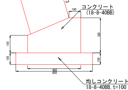
取付工(植生土のう) S=1/50
