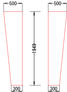
取付工(植生土のう) S=1/50
