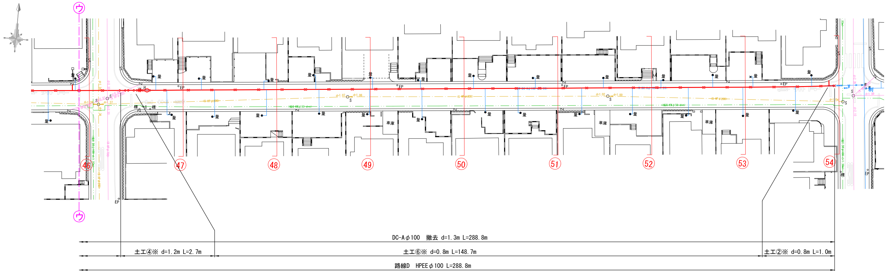
本設平面図-7 S=1 : 500
