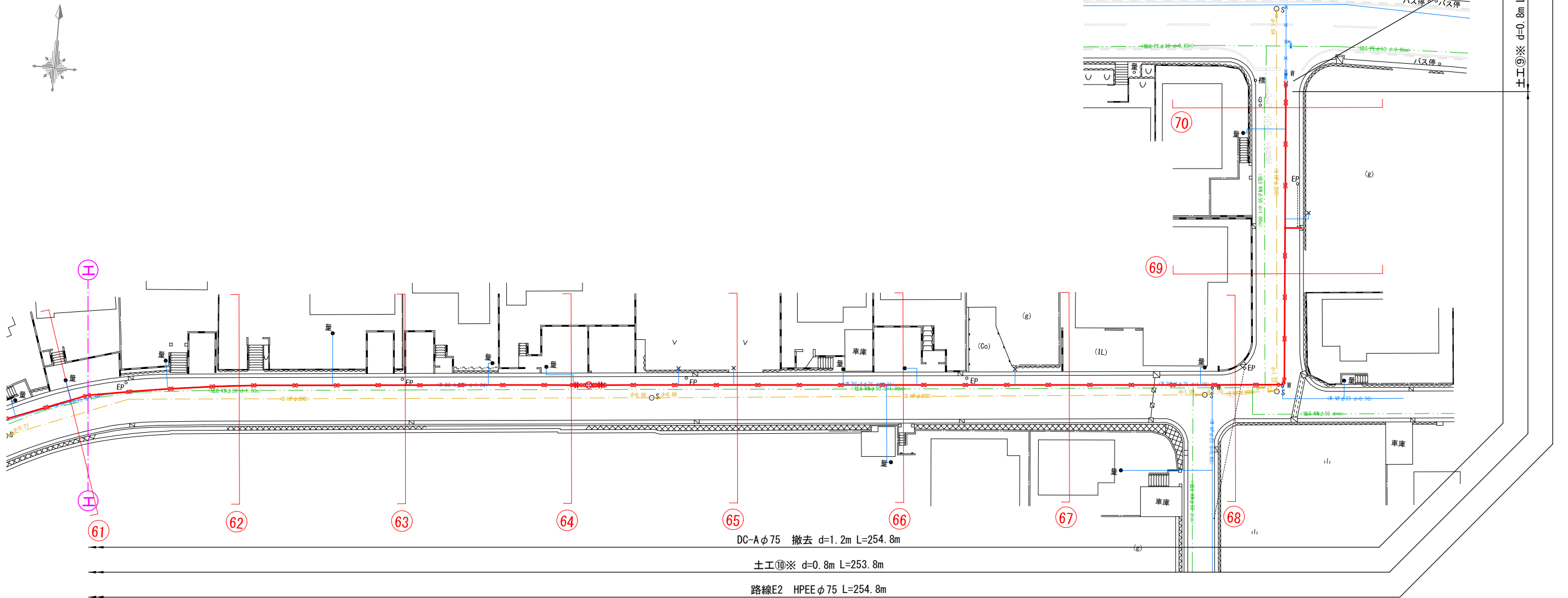
本設平面図-9 S=1 : 500
