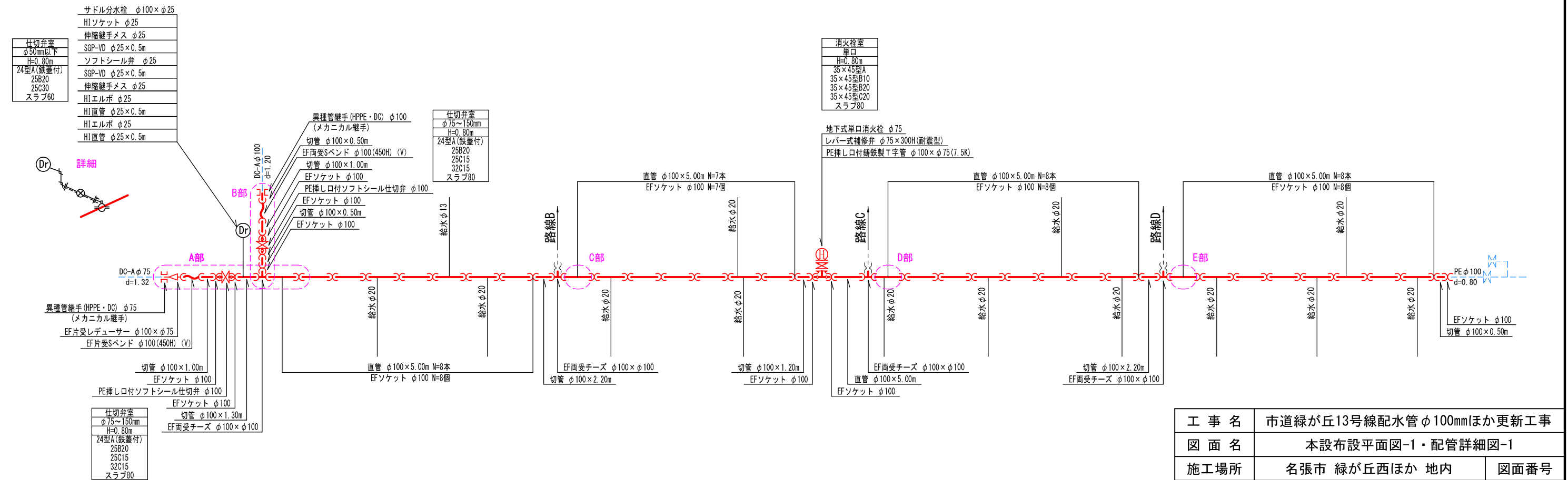
本設配管詳細図-1 S=N0 SCALE
