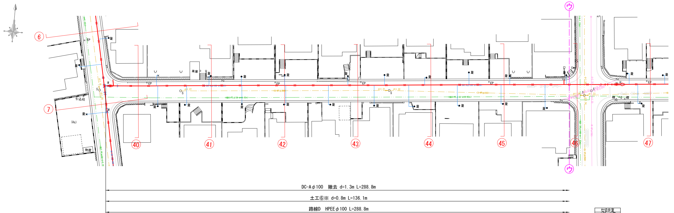
本設平面図-6 S=1 : 500
