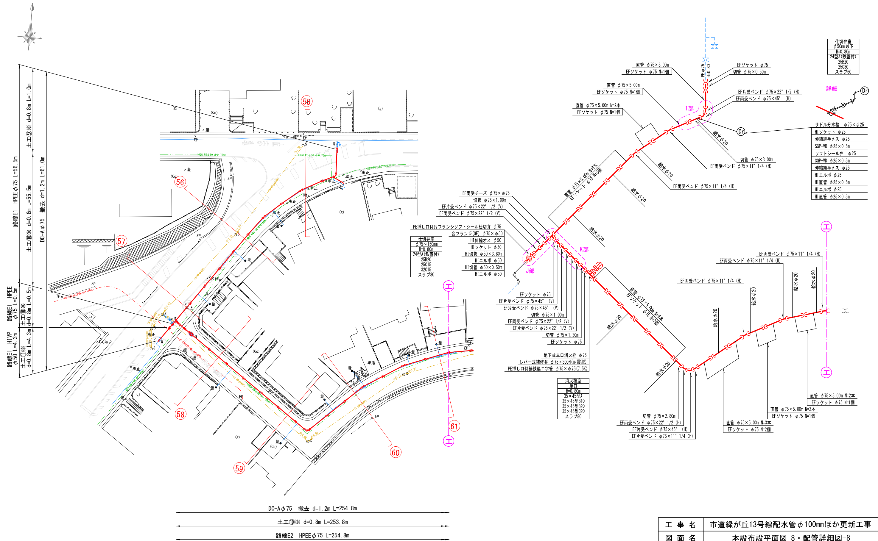
本設平面図-8 S=1 : 500
