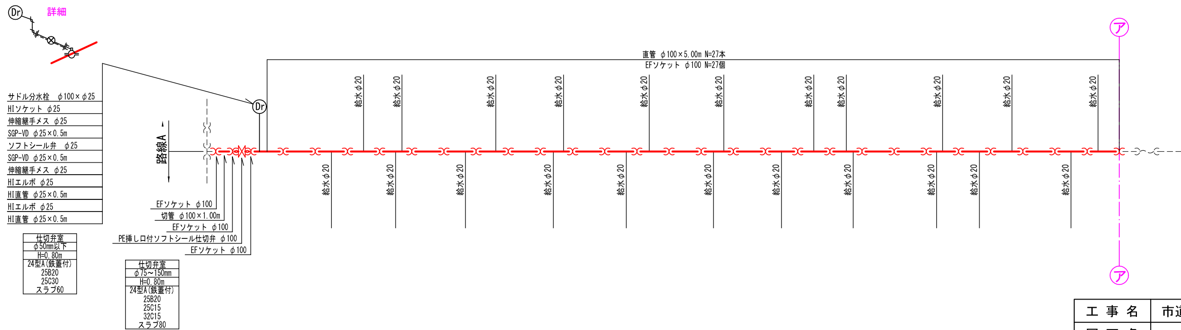
本設配管詳細図-2 S=NO SCALE
