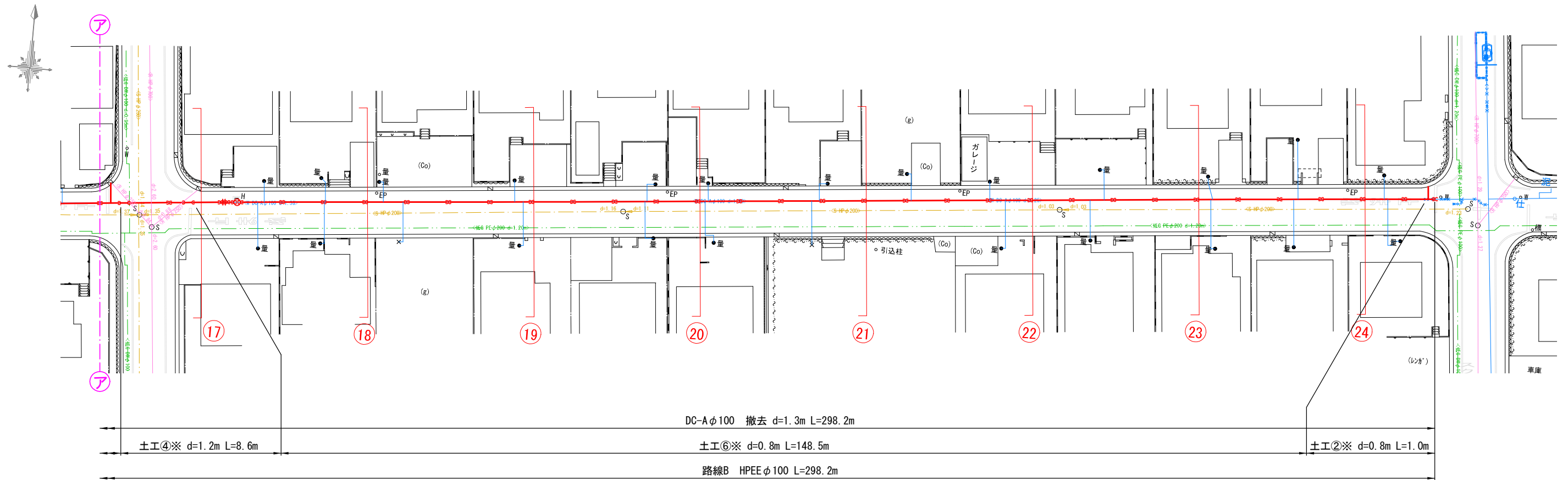
本設平面図-3 S=1 : 500
