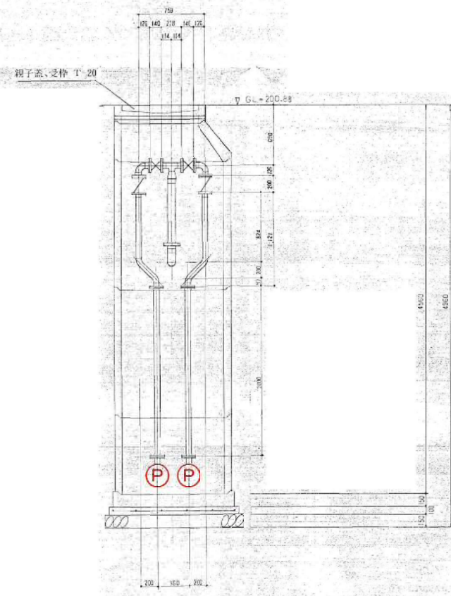
断面図
